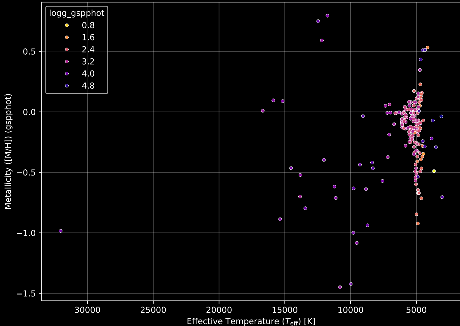
APOGEE DR17 Field: [203+00] Stellar Population Parameters (n= 208)
